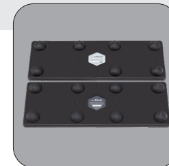
NEQ-K / NEQ-H
